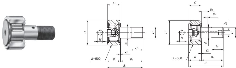
CF...BR Stud dia d_1 3-10mm CF...BR Stud dia d_1 12-30mm
